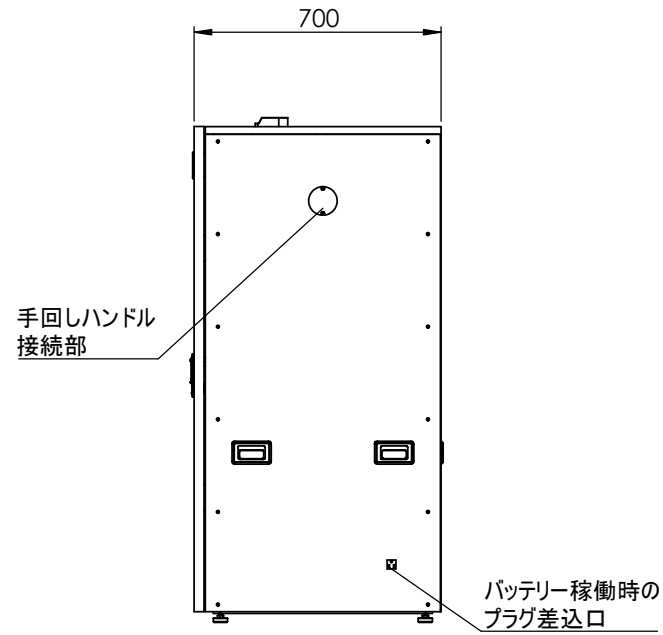
右側面図
