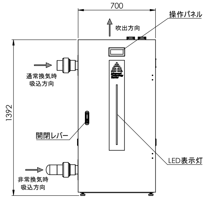
正面図
